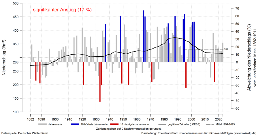
Entwicklung des Niederschlags im hydrologischen Winter (Nov-Apr) im Rhein-Lahn-Kreis im Zeitraum 1882 bis 2023
