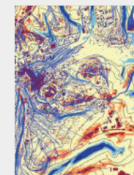
Kaltluftsimulationen
