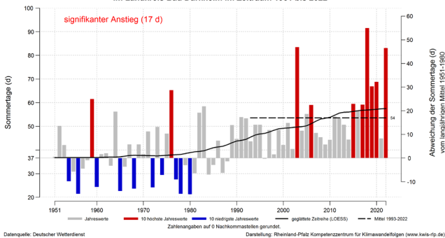
Entwicklung der Sommertage im Kalenderjahr (Jan-Dez) im Landkreis Bad Dürkheim im Zeitraum 1951 bis 2022
