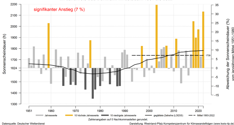
Entwicklung der Sonnenscheindauer im Kalenderjahr (Jan-Dez) im Landkreis Bad Dürkheim im Zeitraum 1951 bis 2022
