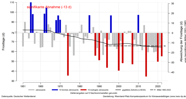
Entwicklung der Frosttage im Kalenderjahr (Jan-Dez) im Landkreis Bad Dürkheim im Zeitraum 1951 bis 2022
