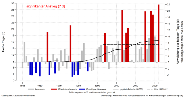
Entwicklung der heißen Tage im Kalenderjahr (Jan-Dez) im Landkreis Bad Dürkheim im Zeitraum 1951 bis 2022
