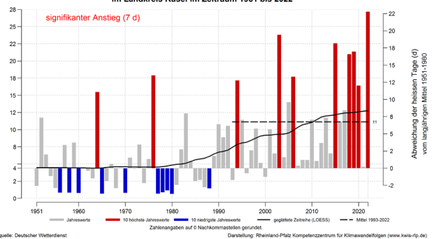
Entwicklung der heißen Tage im Kalenderjahr (Jan-Dez) im Landkreis Kusel im Zeitraum 1951 bis 2022
