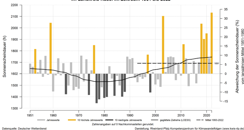
Entwicklung der Sonnenscheindauer im Kalenderjahr (Jan-Dez) im Landkreis Kusel im Zeitraum 1951 bis 2022
