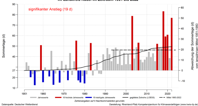
Entwicklung der Sommertage im Kalenderjahr (Jan-Dez) im Landkreis Kusel im Zeitraum 1951 bis 2022
