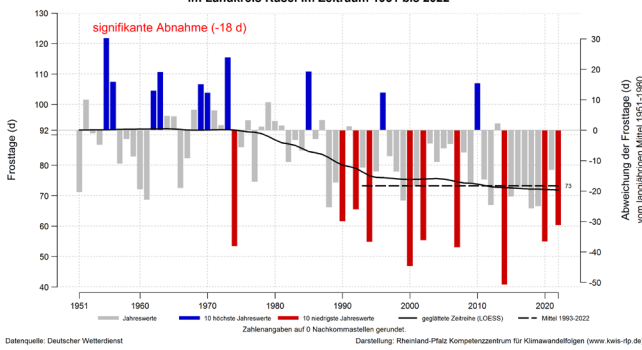
Entwicklung der Frosttage im Kalenderjahr (Jan-Dez) im Landkreis Kusel im Zeitraum 1951 bis 2022
